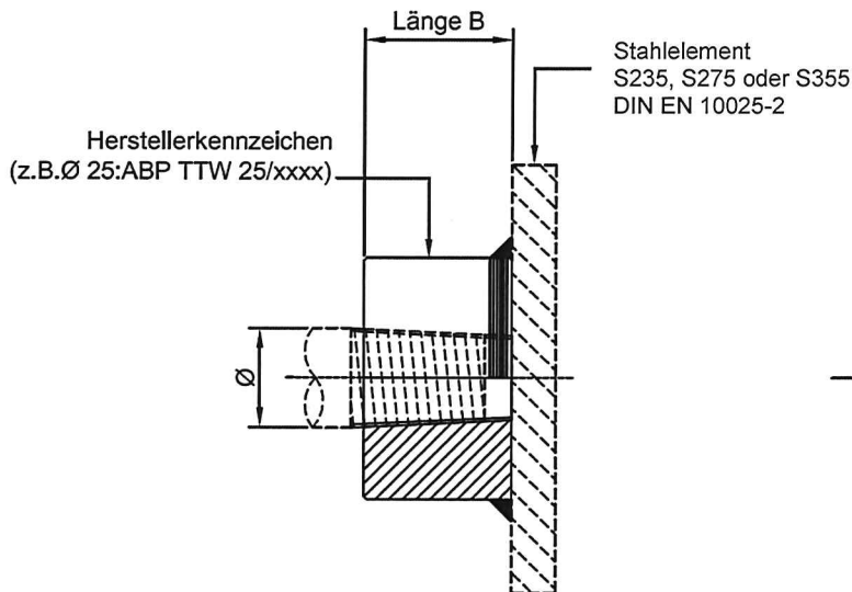
Ansicht Anschweissmuffe TTW
